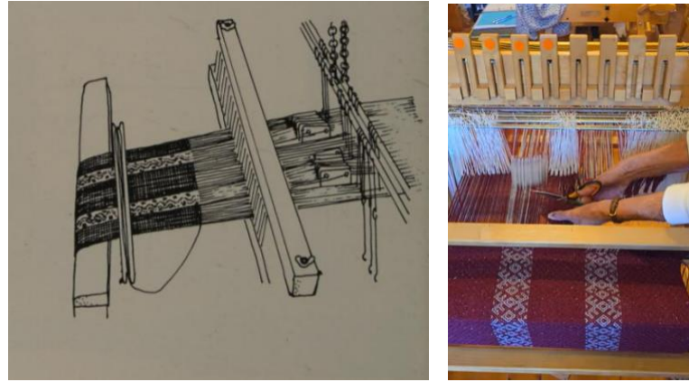
Görsel 11. Tablet (çarpana) dokuma ile konvansiyonel dokumanın aynı tezgâh üzerinde birlikte uygulanışını gösteren şematik çizim (Sutton ve Holtom, 1975: 98), uygulama örneği URL 3
