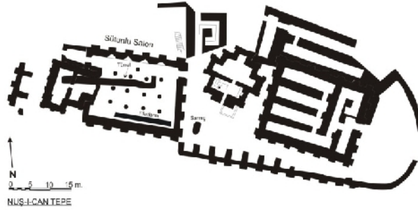
Çizim-2: Nuş-i Can Tepe Mimari Plan ve Sütunlu Salon
