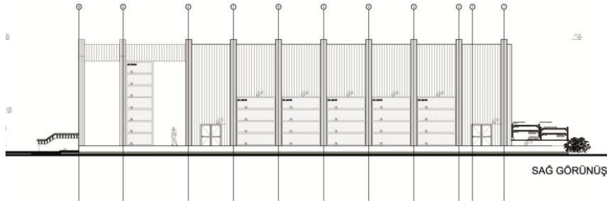
Şekil 16. Kapalı spor salonu sağ görünüş, Çelik, 2017
