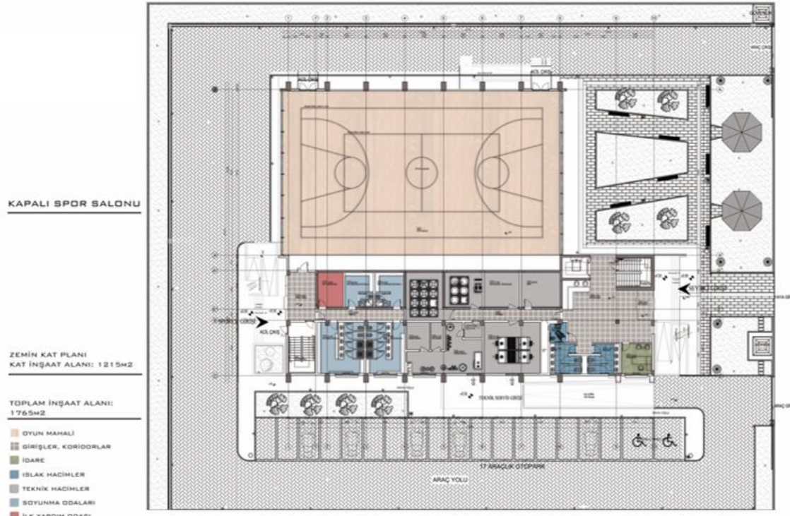
Şekil 8. Kapalı spor salonu zemin kat planı (Çelik, 2017)
